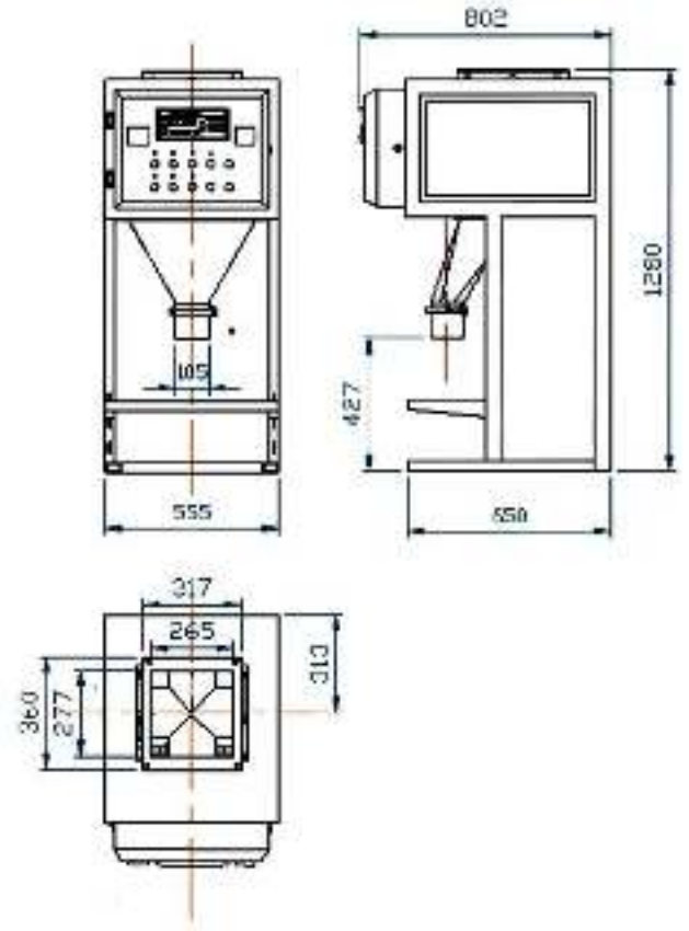
MACHINE DIMENSION ขนาดตัวเครื่อง
